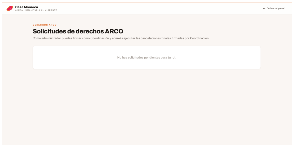
Figura 3.9: Bandeja del panel de administración para la gestión, dictamen e histórico de Solicitudes ARCO.
