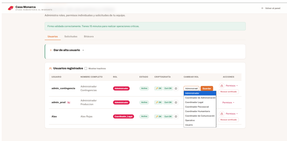
Figura 3.3: Menú desplegable con las 8 jerarquías de control de acceso basado en roles (RBAC) del sistema.
